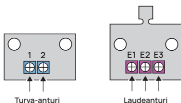
Kuva 3. Turva-/laudeanturin asennus.
