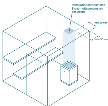
Abbildung 4. Sicherheitssensor installieren: stehender Saunaofen.
