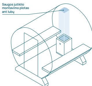
11 pav. Saugos jutiklio montavimas ant lubų statinės tipo pirtyse: ant grindų montuojamas šildytuvas.
