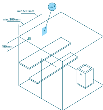
Figur 8. Bänksensorns placering från hörn, öppning och tak
