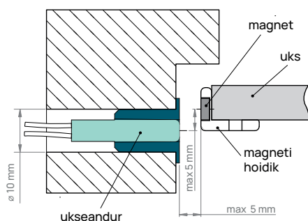
Joonis 2. Ukseanduri paigaldus.
