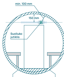
13 pav. Sumontuokite suoliuko jutiklį statinės tipo pirtyje ant apskritos sienos, priešingoje pusėje nei šildytuvus.
