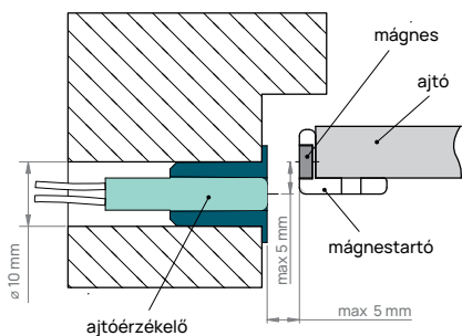
2. ábra Az ajtóérzékelő elhelyezése.
