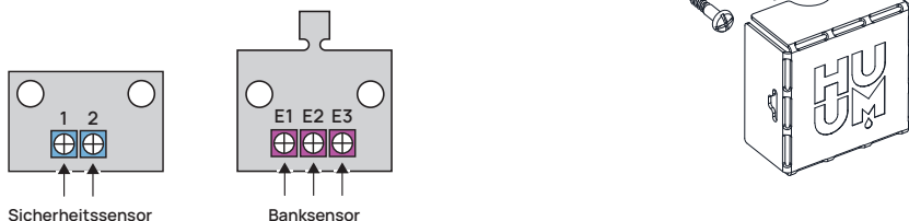
Abbildung 3. Einbau Sicherheits-/Banksensor.
