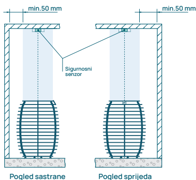
Slika 4 Instaliranje sigurnosnog senzora: podna grijalica.
