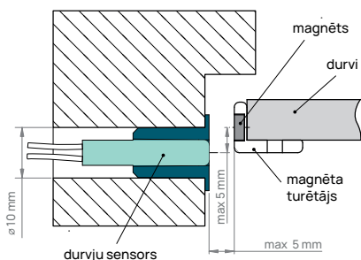
2. attēls. Durvju sensora novietojums.
