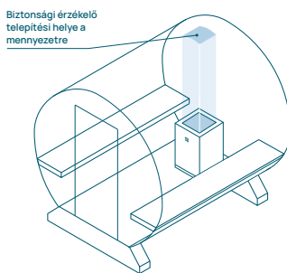
11. ábra A biztonsági érzékelő mennyezetre történő telepítése hordószaunákban: padlóra szerelt fűtőberendezés
