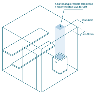
4. ábra A biztonsági érzékelő telepítése: padlóra szerelt fűtőberendezés.
