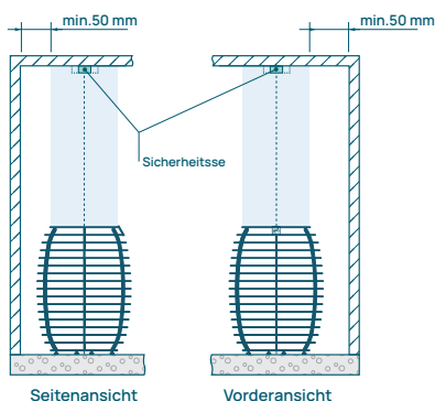
Abbildung 4. Sicherheitssensor installieren: stehender Saunaofen.
