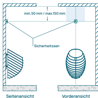
Abbildung 5. Sicherheitssensor an der Wand montieren: wandmontierter Saunaofen
