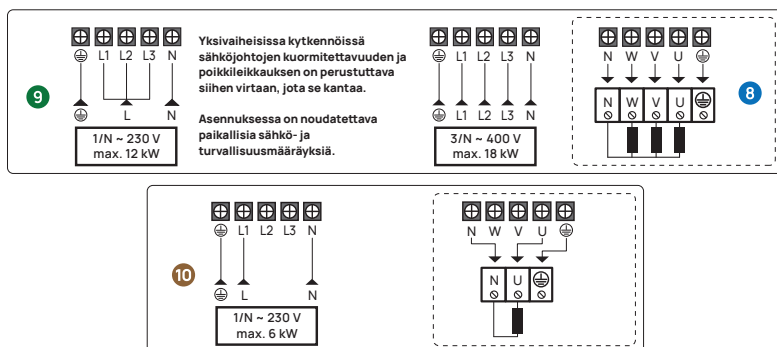
Kuva 1. Kiukaan sähköliitännät.
