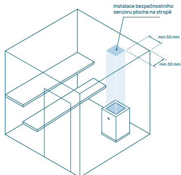
Obrázek 4. Instalace bezpečnostního senzoru: ohřívač montovaný k podlaze.
