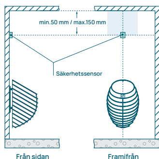
Figur 5. Installera säkerhetssensorn på väggen: väggmonterat bastuaggregat
