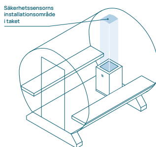
Figur 11. Installation av säkerhetssensor i taket i bastutunna: golvmonterat bastuaggregat.
