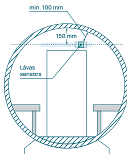
13. attēls. Uzstādiet lāvas sensoru pirts pirts mucā uz apalās gala sienas, pretējā pusē krāsnij.
