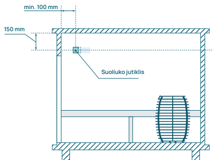
12 pav. Sumontuokite suoliuko jutiklį statinės tipo pirtyje ant išlenktos sienos, priešingoje pusėje nei šildytuvus.
