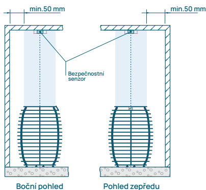
Obrázek 4. Instalace bezpečnostního senzoru: ohřívač montovaný k podlaze.
