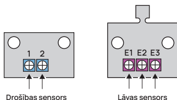
3. attēls. Drošības/lāvas sensora uzstādīšana.
