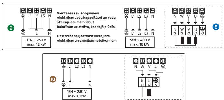
1. attēls. Krāsns elektriskie savienojumi.
