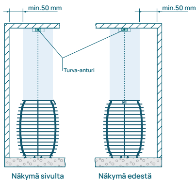
Kuva 4. Turva-anturin asennus: lattiaan asennettava kiuas.
