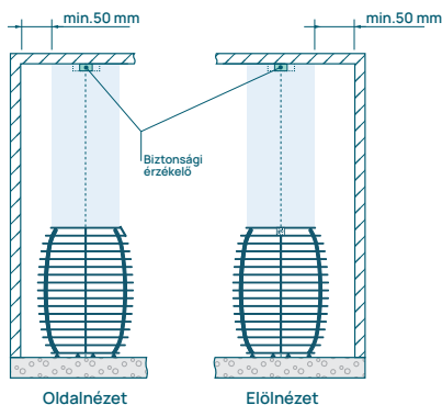
4. ábra A biztonsági érzékelő telepítése: padlóra szerelt fűtőberendezés.
