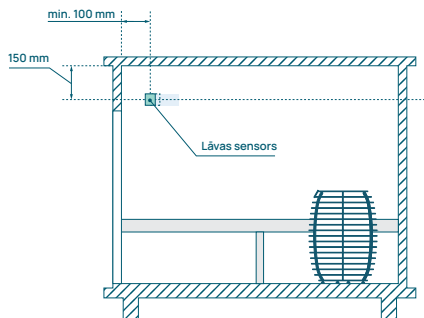
12. attēls. Uzstādiet lāvas sensoru pirts mucā pie ieliktās sienas, pretējā pusē krāsnij.
