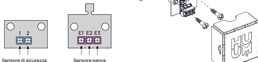
Figura 3. Installazione sensore di sicurezza/panca.
