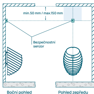
Obrázek 5. Instalace bezpečnostního senzoru na stěnu: nástěnný ohřívač
