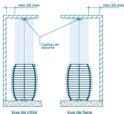
Figure 4. Installation du capteur de sécurité : chauffage au sol.
