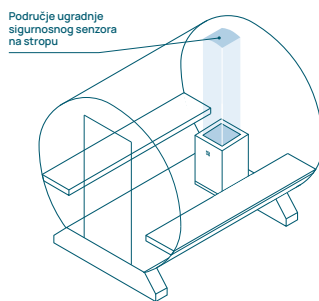
Slika 11 Instaliranje sigurnosnog senzora na strop u bačvastim saunama: podna grijalica.
